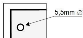
Detalhe do furo de fixação
